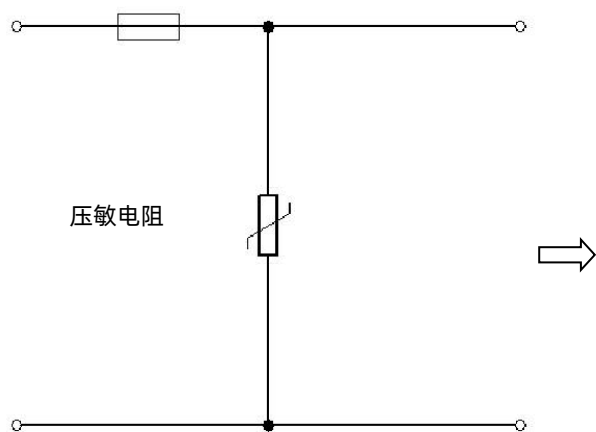
图a 电涌保护典型电路
