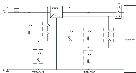
光伏逆变器
