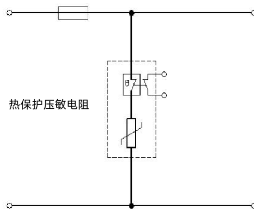
图b 电涌保护高可靠性电路
