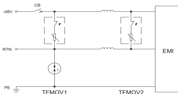
射频拉远单元（直流型）
